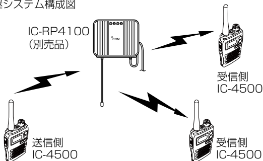
中継システム構成図
